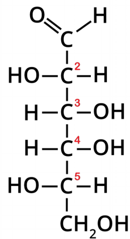
L-Galactose
