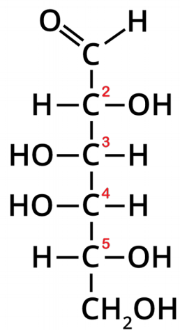
D-Galactose
