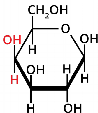
Galactose
